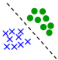
Linear separability
